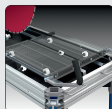
Fűrészkosci 6 kerékkel
